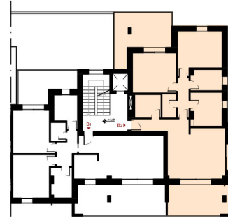
KEY-PLAN PIANO PRIMO scala 1:500
